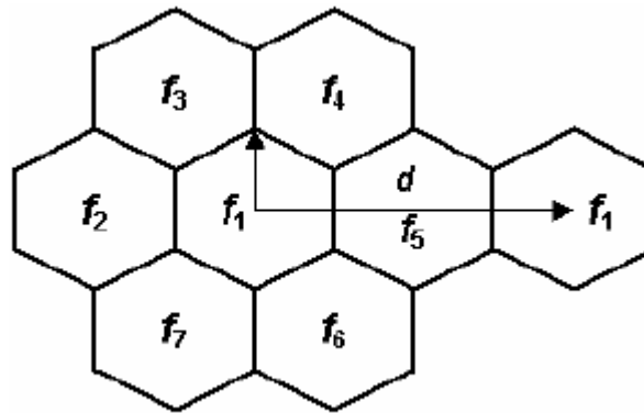
Figure 15 : Réseau cellulaire.
