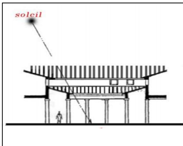
Fig.16. Coupe d'un Patio à Rome
