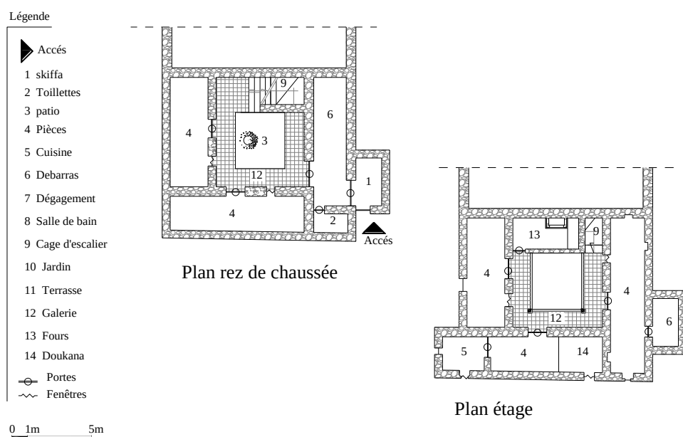
Fig.40. Plan d'une habitation traditionnelle à patio de vieux Mila 01.
