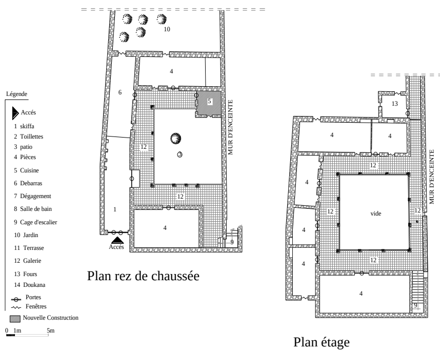
Fig.41. Plan d'une habitation traditionnelle à patio de vieux Mila 02.
