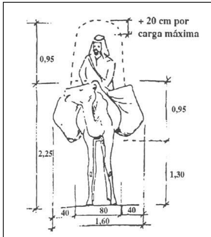
Fig.17. Les dimensions horizontale et verticale pour le passage d'un chameau chargé.
