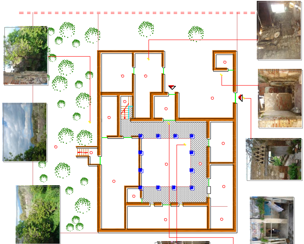
PLAN REZ DE CHAUSSEE
