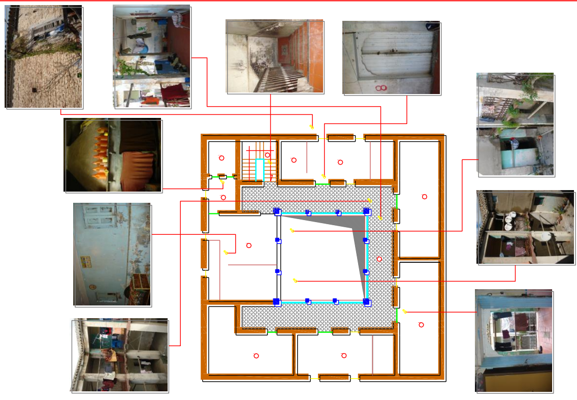
PLAN ETAGE
